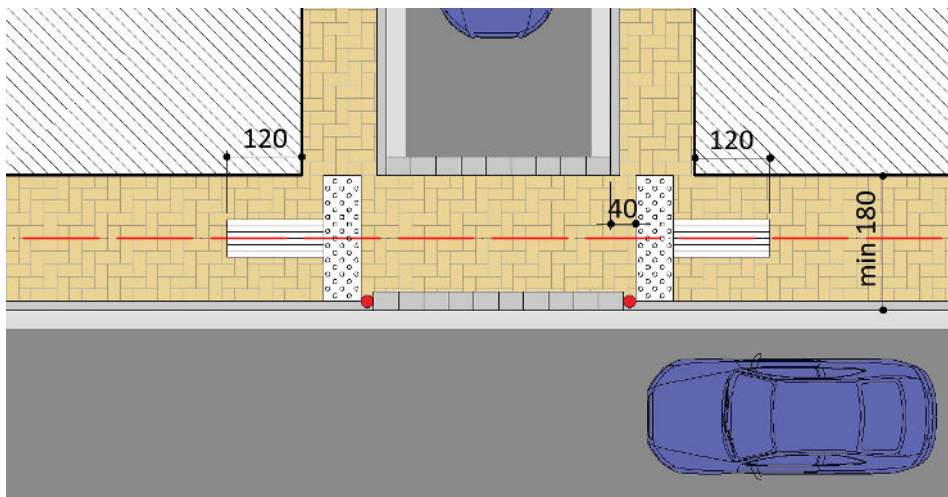
Principe d'aménagement du dispositif podotactile d'un trottoir traversant d'une largeur supérieure ou égale à 180 cm
